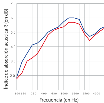
— Tabique 78/48 Placo® Phonique 15* con Supralaine R_w = 49 (-5;-12) R_A = 45,2 — Tabique 78/48 Estándar 15** con Supralaine R_w = 45 (-2;-9) R_A = 43
