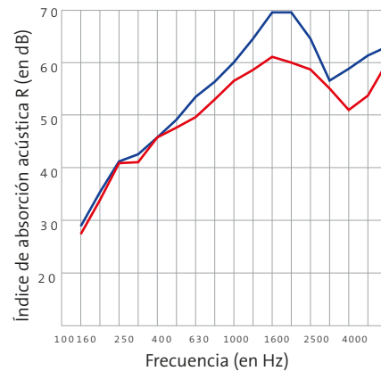
— Tabique 98/48 Placo® Phonique 13* con Placover R_w = 55 (-3;-8) R_A = 53,1 — Tabique 98/48 Estándar 13** con Placover R_w = 54 (-3;-8) R_A = 51,9
